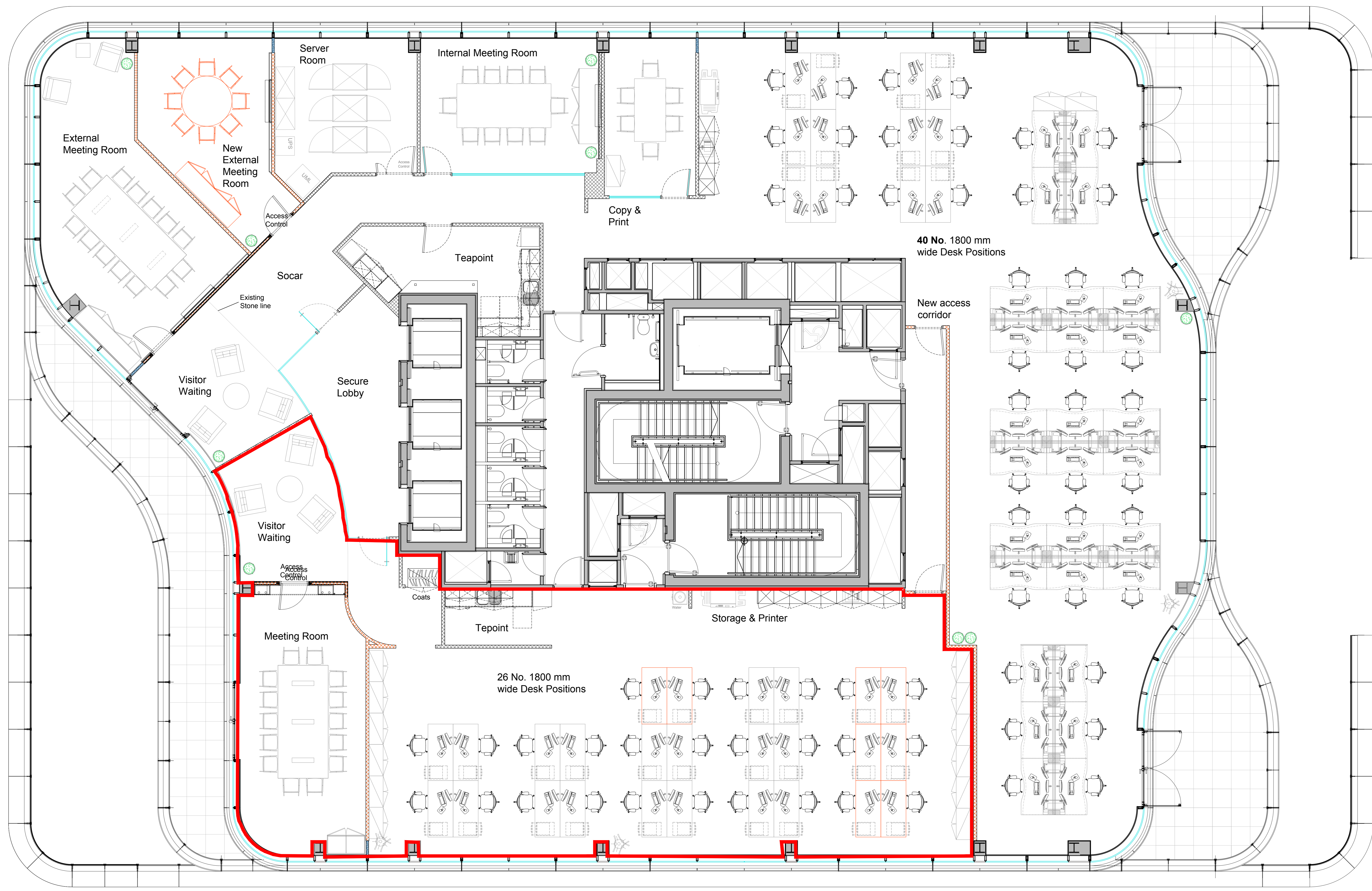
2 Layout 02 Scale: 1:50
